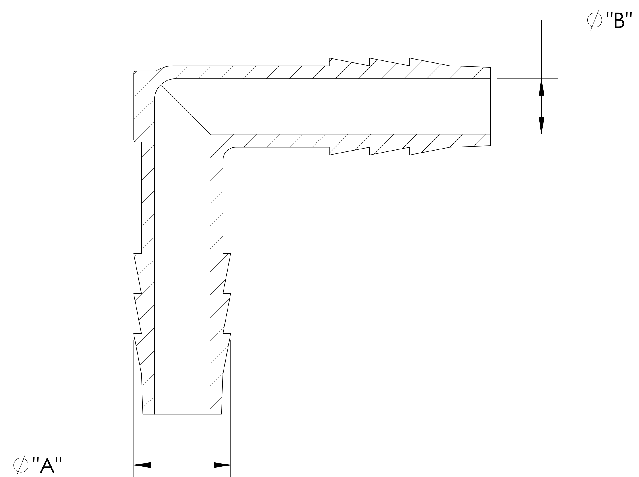
SECTION A-A
