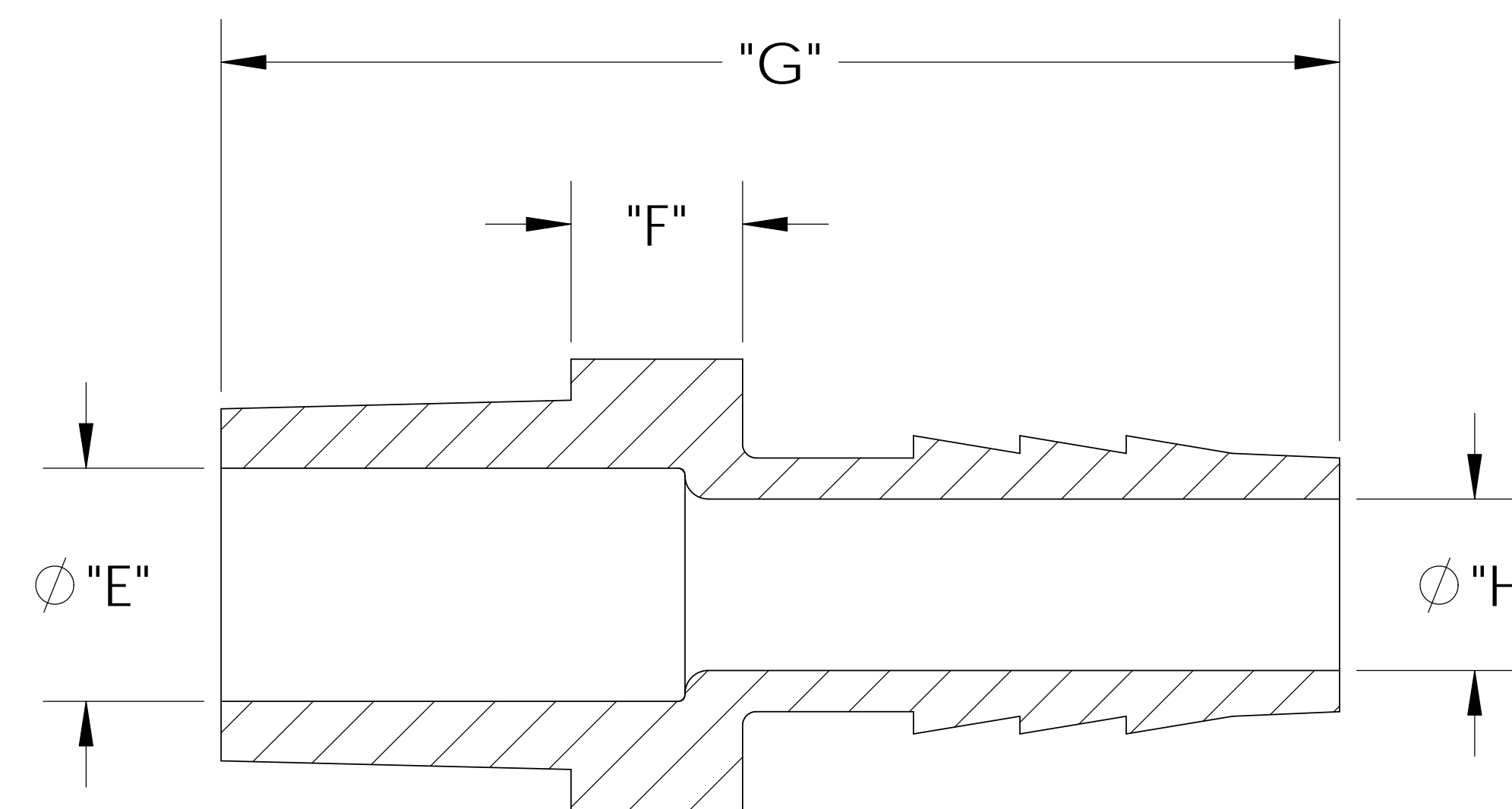
SECTION A-A
